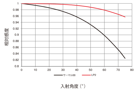
感度 vs 入射角
