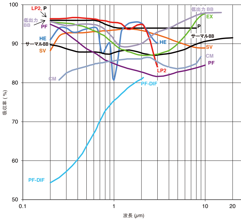
吸収率 vs 測定波長
