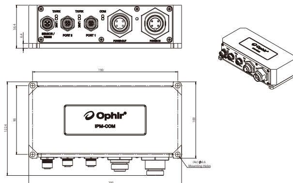
IPM-COM-EtherNet/IP-M (M12, Mini 7/8")
