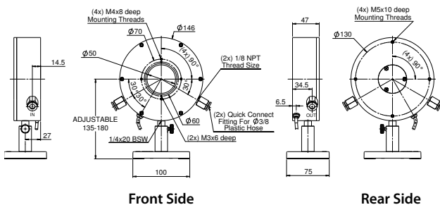
5000W-BB-50 / 5000W-LP2-50
